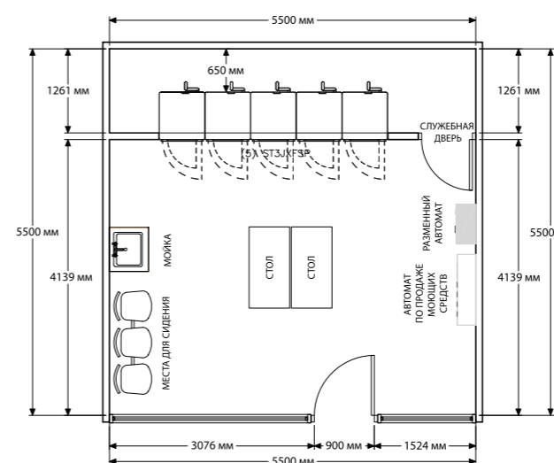
Схема расположения оборудования
